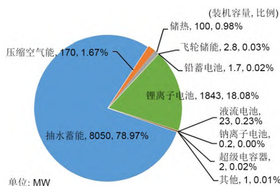
图4 2021年中国储能新增装机容量
