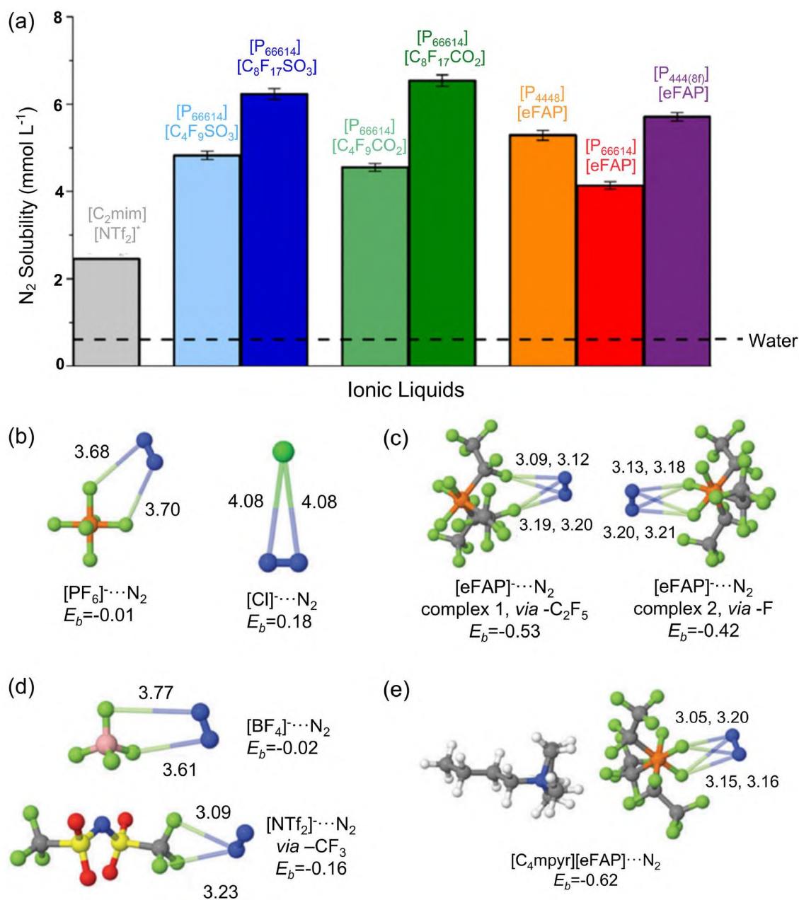
图 4 (网络版彩色) 离子液体结构对 N 2 溶解度的影响. (a) N 2 在不同离子液体中的溶解度 [25] . (b)~(e) 离子液体与 N 2 相互作用示意图 [11]
